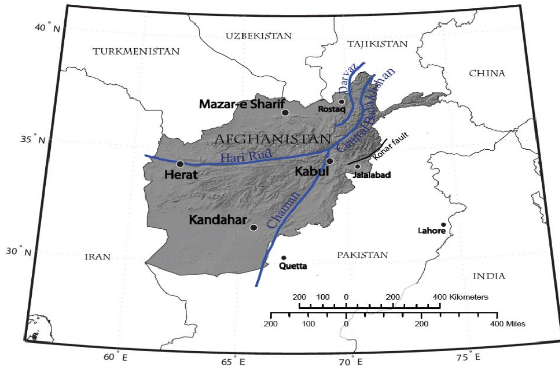
شکل 5. موقعیت چهار شکست عمده در افغانستان (خط های بزرگ آبی)
