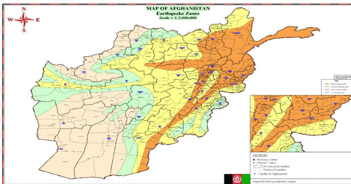
شکل 3. نقشه زمین لرزه خیزی در افغانستان
