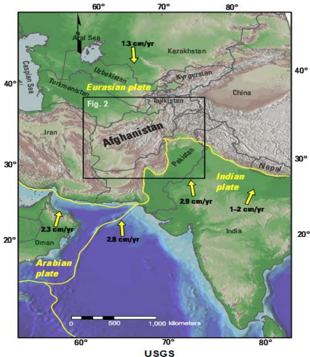
شکل ۲، سرعت حرکت صفحات هند، عرب و اروپایی-آسیا
